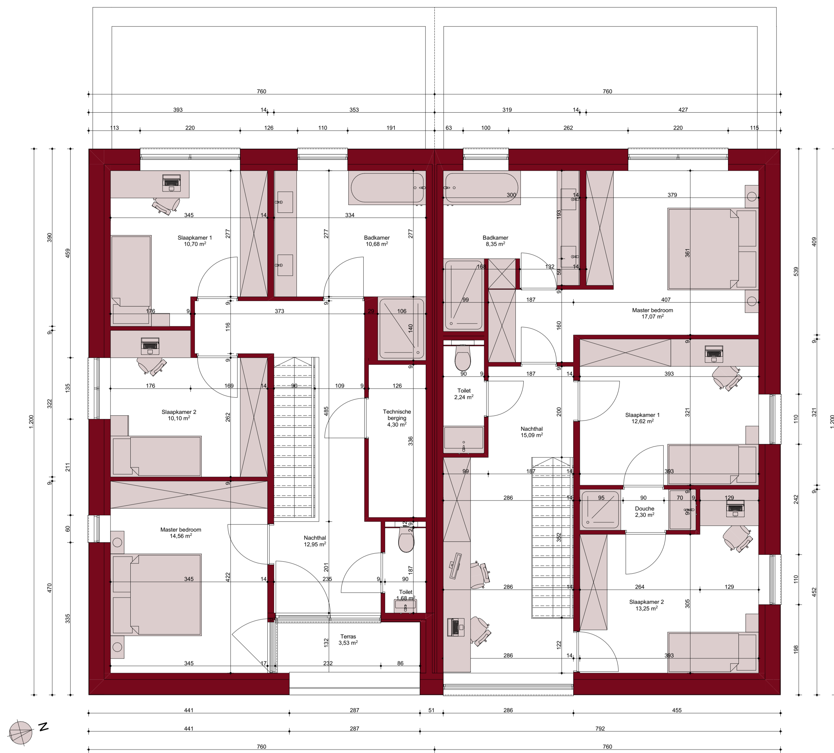
GRONDPLAN VERDIEPING +1/50
