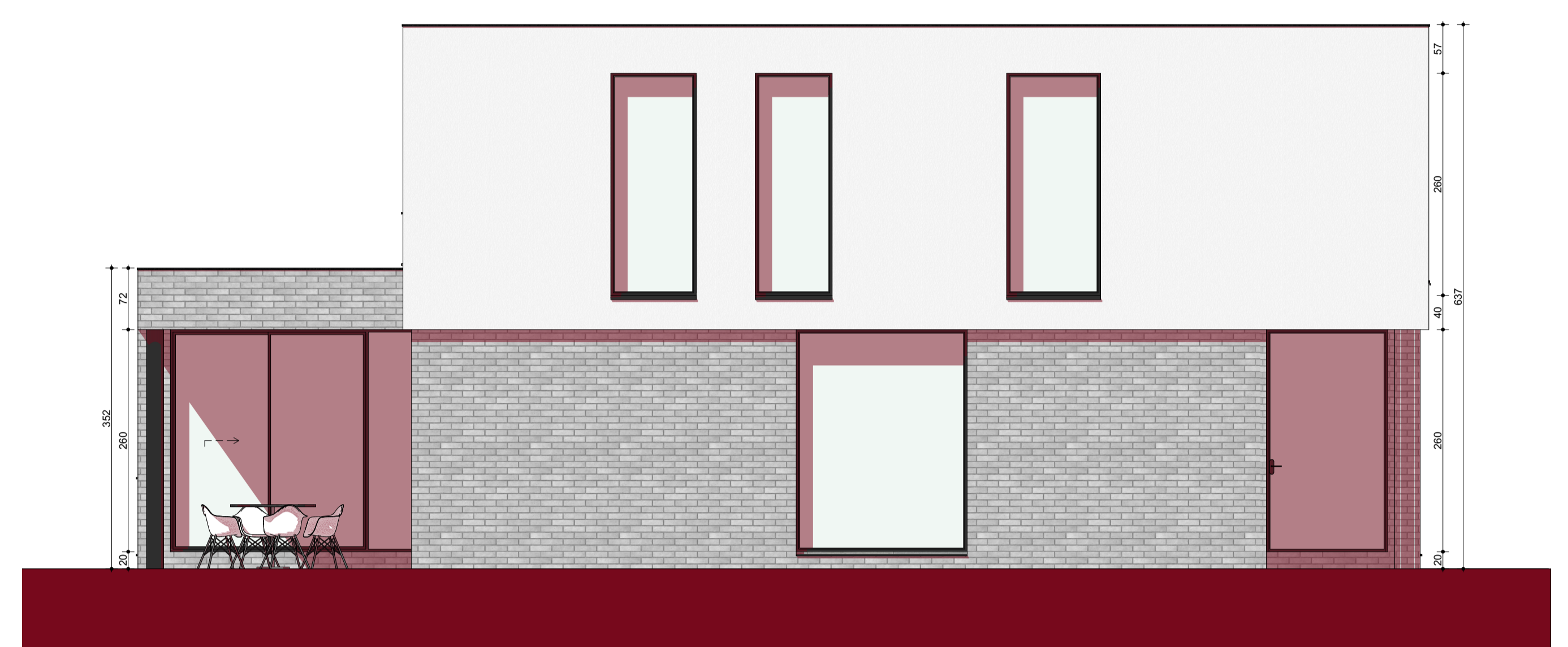
GEVEL LINKS
