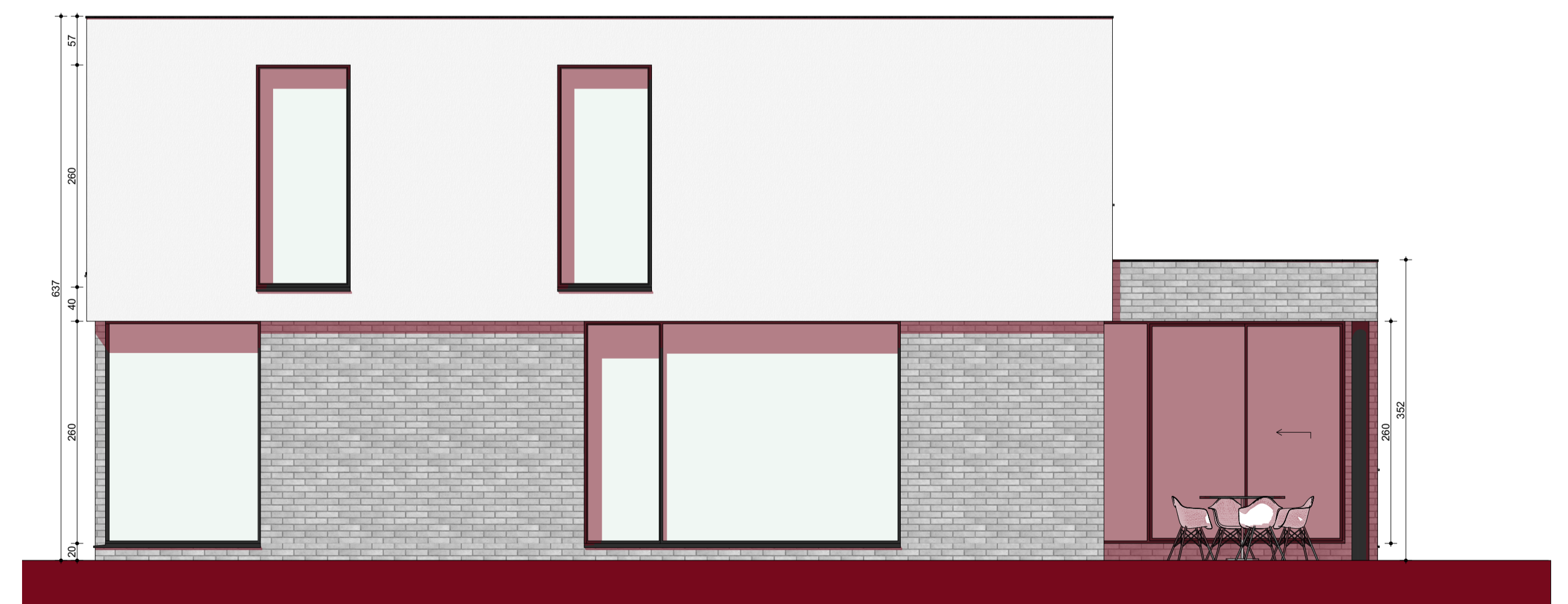
GEVEL RECHTS
