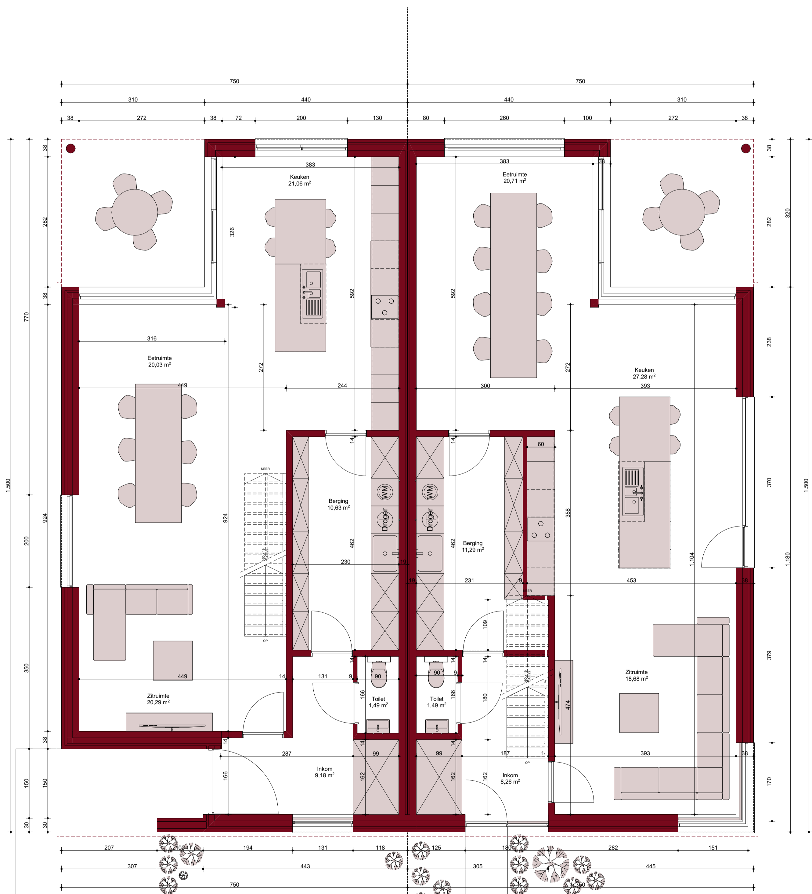
GRONDPLAN GELIJKVLOERS 1/50
