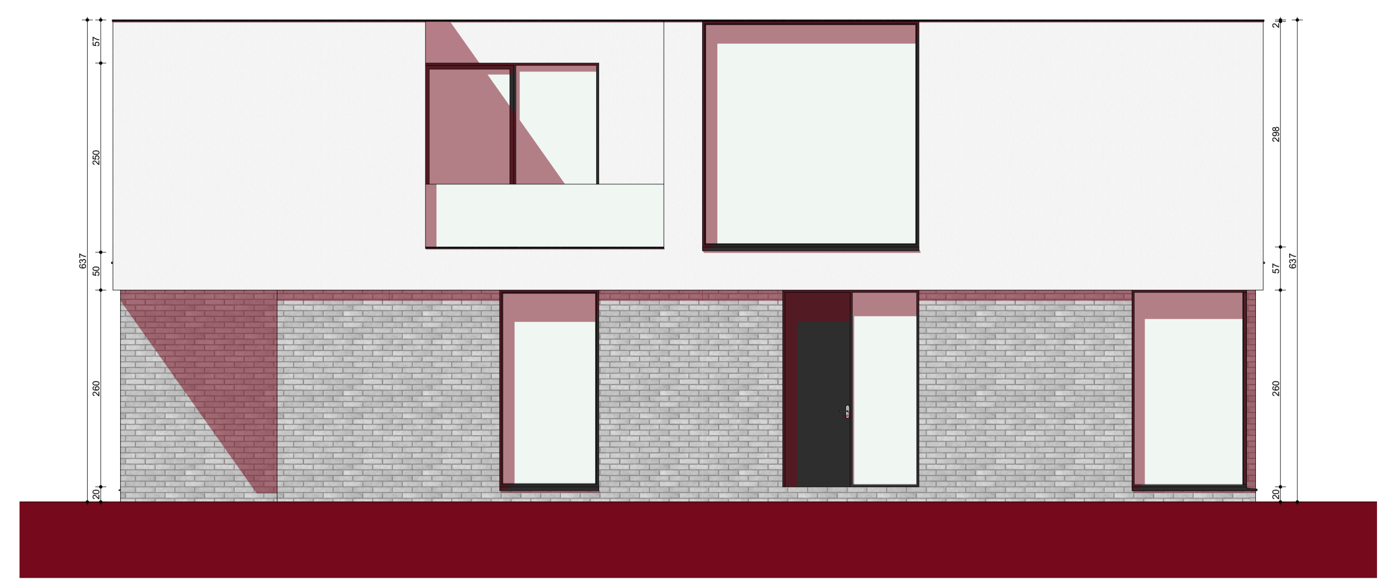
GEVEL VOOR
